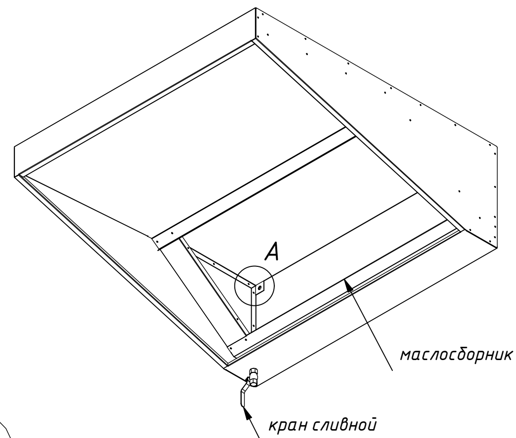
Вид снизу ( 1 : 12 )
