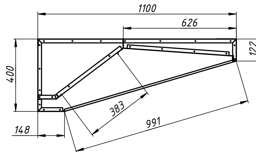
B-B ( 1 : 12 )
